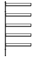
Extension 900 system H1940 W940 D260 H76.3" W37" D10.2"
